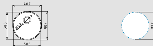
Aufrässhablone beiliegend
