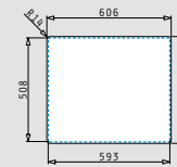
Flächenbündiger Einbau
