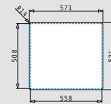
Flächenbündiger Einbau
