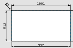
Flächenbündiger Einbau
