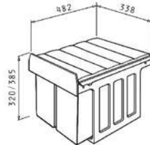
2-fach Trennung Abmessungen: 338 x 320 x 485 mm
