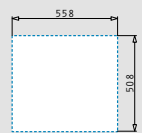
Einbau
