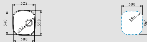
Aufrässhablone beiliegend
