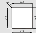
Flächenbündiger Einbau
