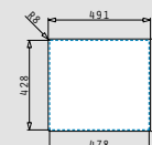
Ausfrässhablone beiliegend
